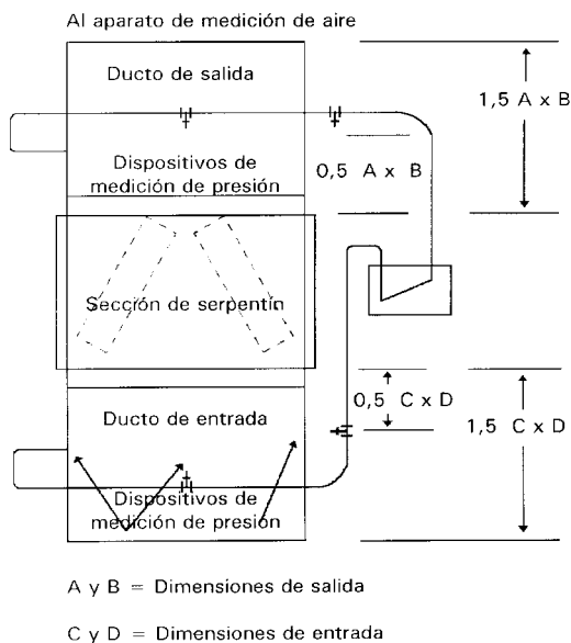
FIGURA 8. Medición de caída de presión estática del aire para una sección de serpentín sin ventiladores
