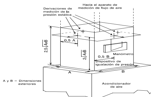
FIGURA 7. Medición de la presión estática externa
