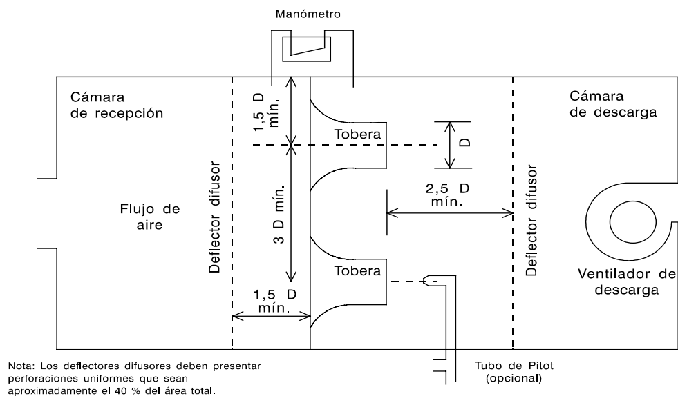
FIGURA 5. Aparato de medición de flujo de aire
