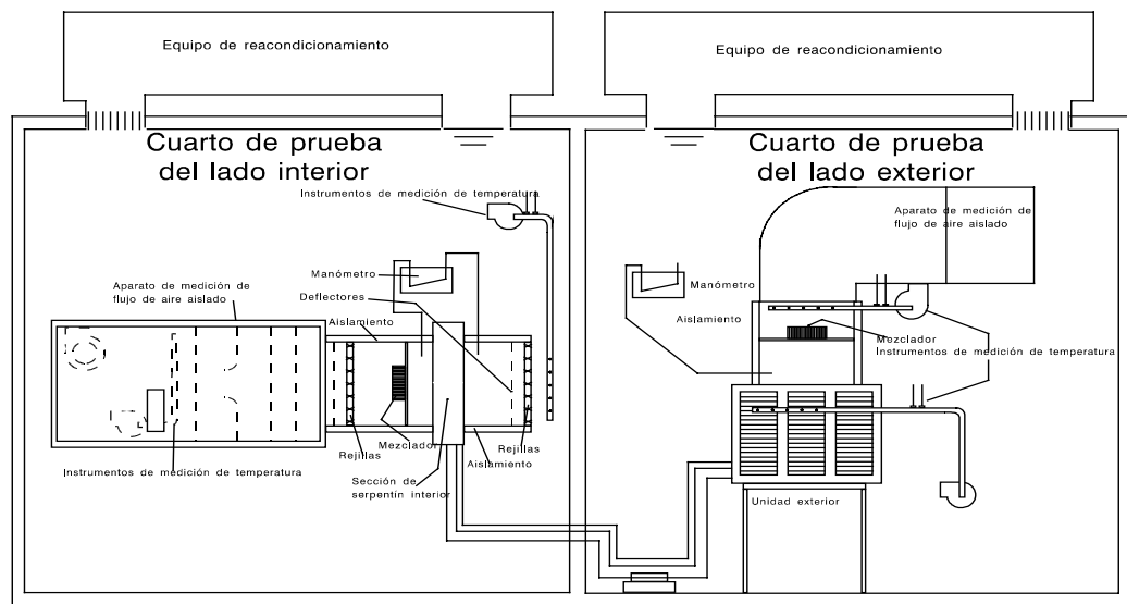
FIGURA 1. Método de túnel aire-entalpía
