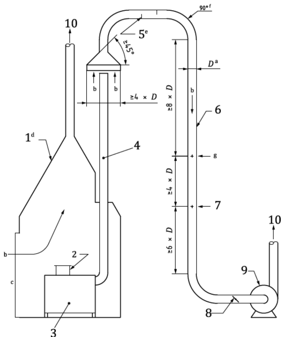
Figura D.2 – Campana y aparatos del túnel de dilución para recolectar emisiones fugitivas (intramuros) de estufas
