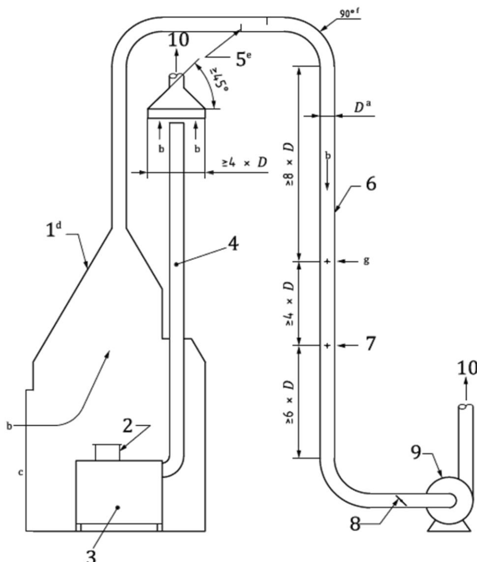
Figura D.1 – Campana y aparatos del túnel de dilución para recolectar las emisiones totales de las estufas
