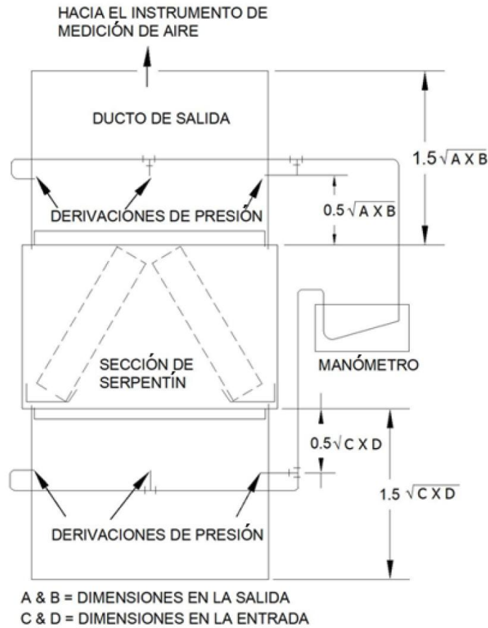
Figura A.8 - Medición de caída de presión estática debido a los serpentes (sin ventilador)
