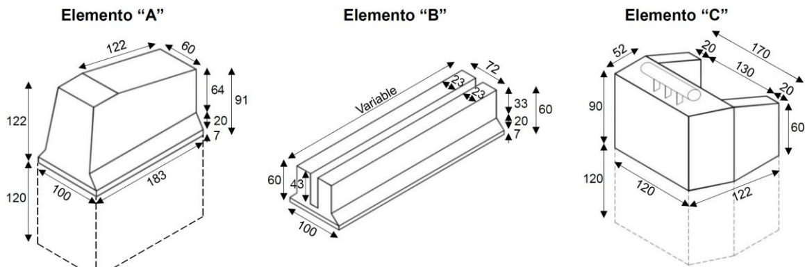
FIGURA 12.- Esquema de los elementos del espolón (isométrico)
