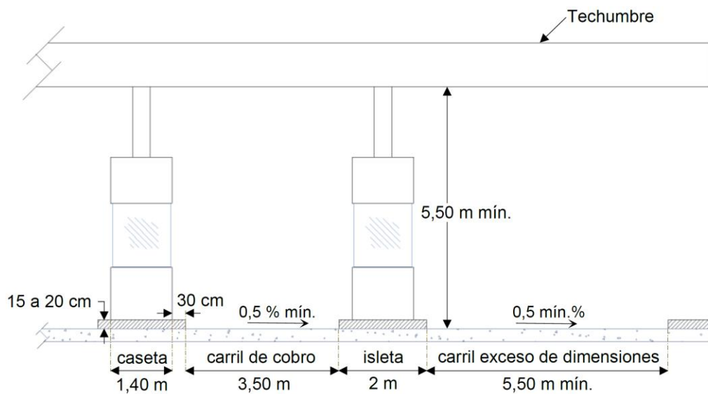
FIGURA 6.- Alzado frontal de las casetas de cobro
