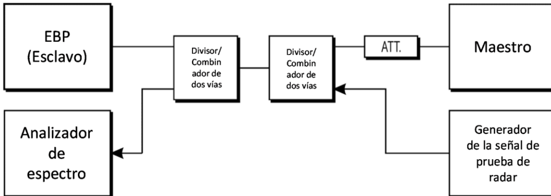
Figura 8. Configuración C.
