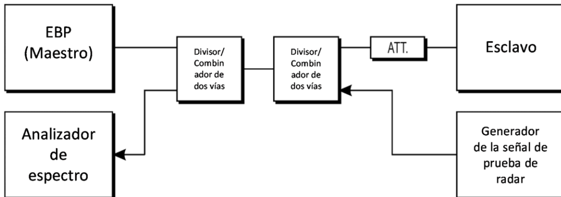
Figura 6. Configuración A.
