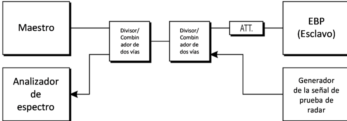
Figura 7. Configuración B.
