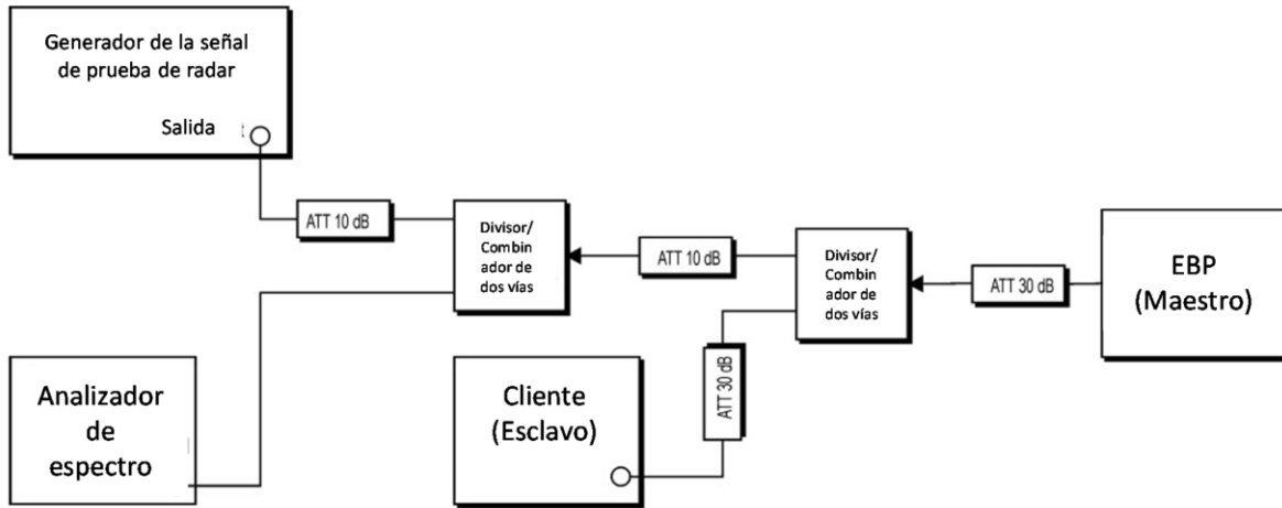
Figura 14. Ejemplo de configuración conducida donde el EBP es un maestro y las formas de onda de prueba de radar se inyectan en el maestro.
