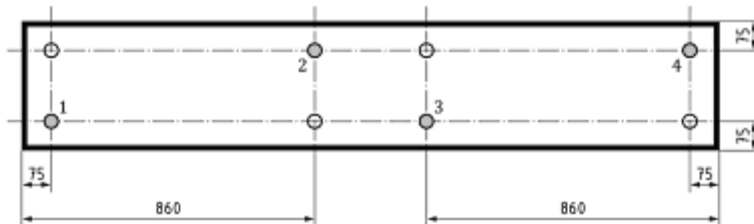
Ilustración 2 - Ubicación de la prueba de arrancamiento en SBD que cubre parcialmente el durmiente o soporte de concreto.
