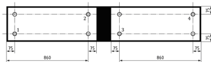
Ilustración 3 - Ubicación de la prueba de arrancamiento en SBD que cubre totalmente la parte inferior del durmiente o soporte de concreto.
