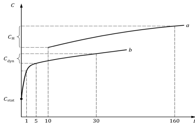
Ilustración 1 - Ejemplo de curva de módulo de asiento dependiente de la frecuencia (con y sin fuerza de precarga).
