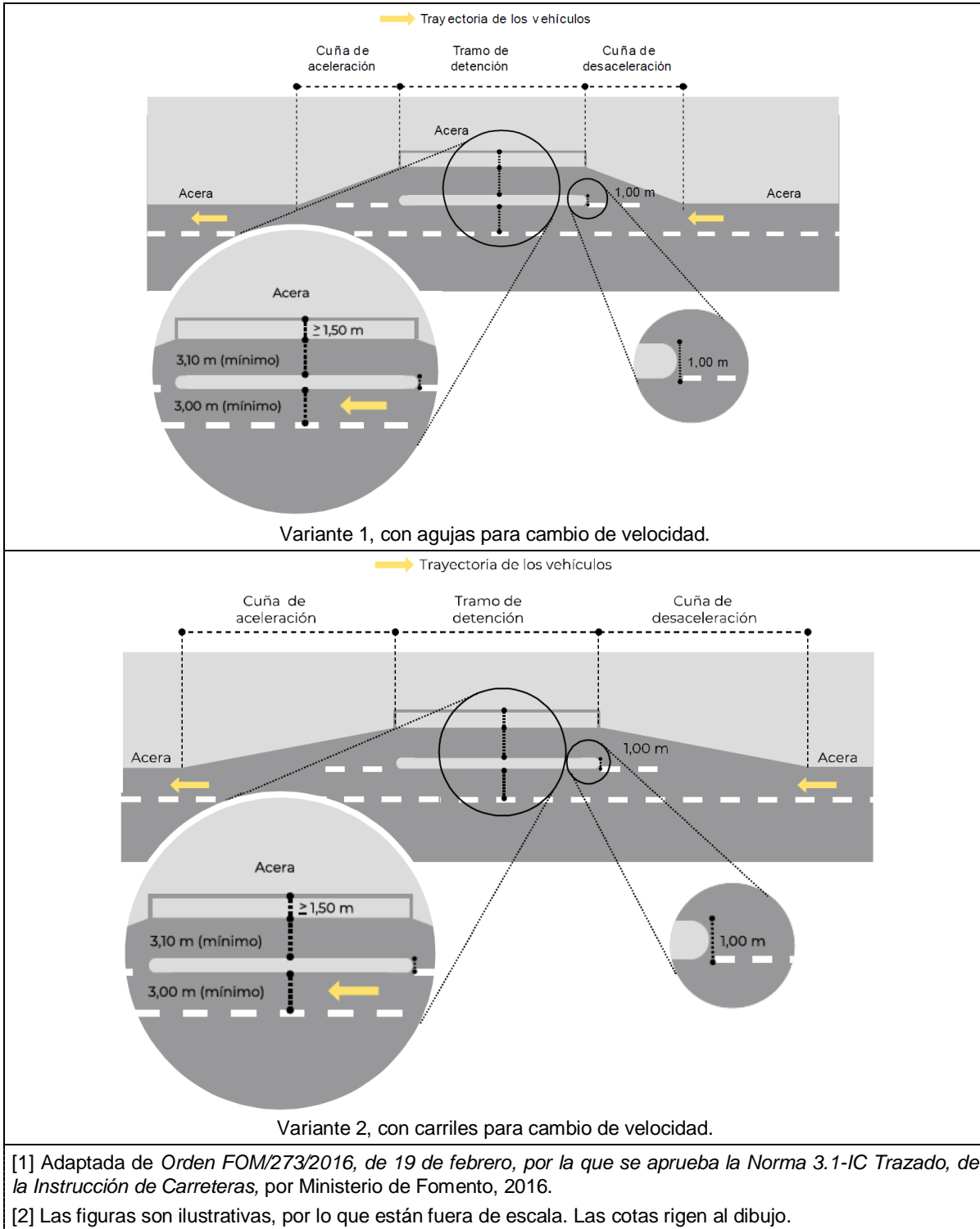
Figura 78.- Paradas de vehículos de transporte público de pasajeros [1] [2]
