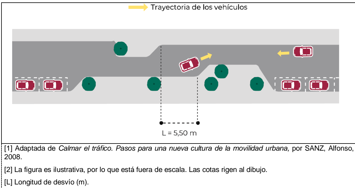
Figura 104.- Zigzag creado por estrechamiento lateral alternativo de la calzada [1] [2]
