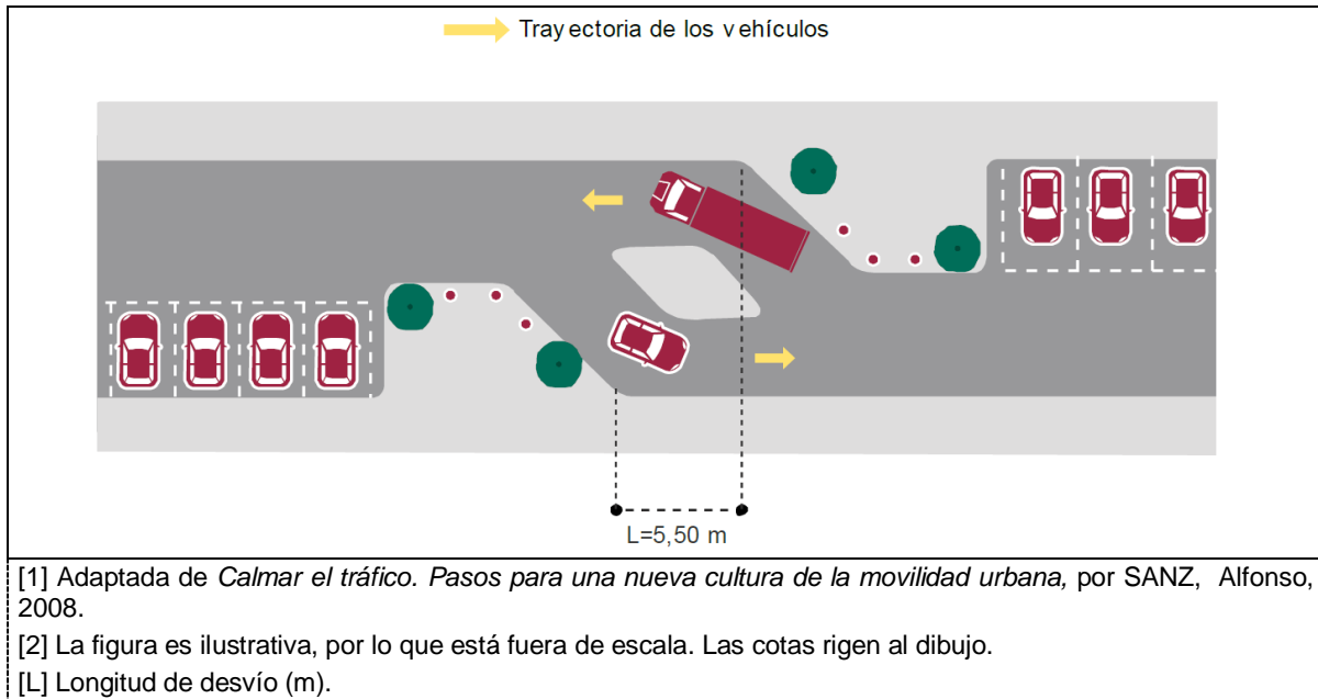
Figura 105.- Zigzag creado por estacionamiento, alternado e isleta central [1] [2]
