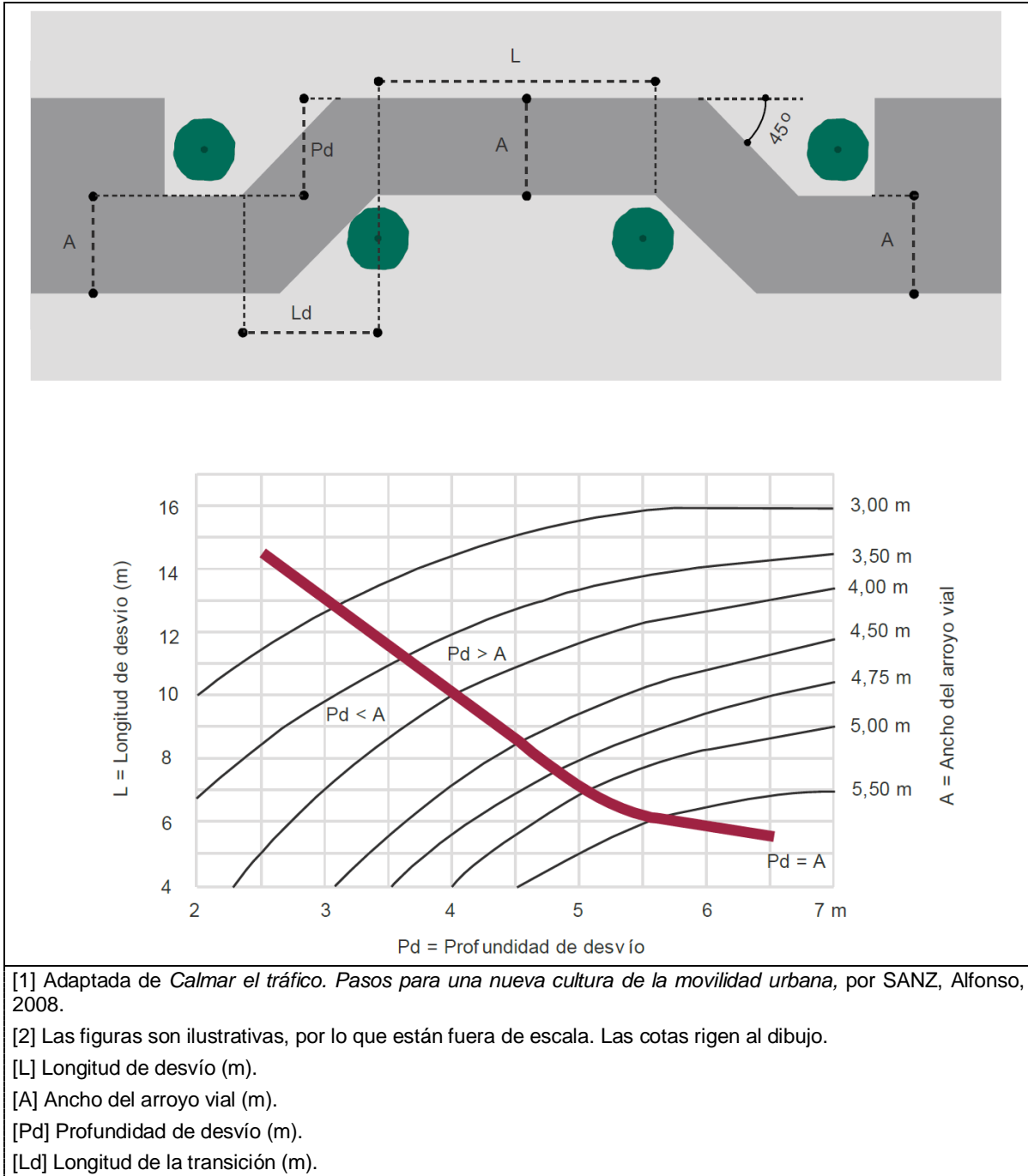
Figura 101.- Dimensionamiento de zigzag [1] [2]
