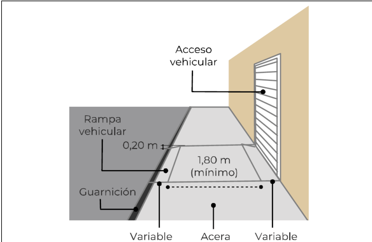
Variante 3, rampa sobre franja de mobiliario o vegetación con desnivel para el acceso en franja de fachada.
