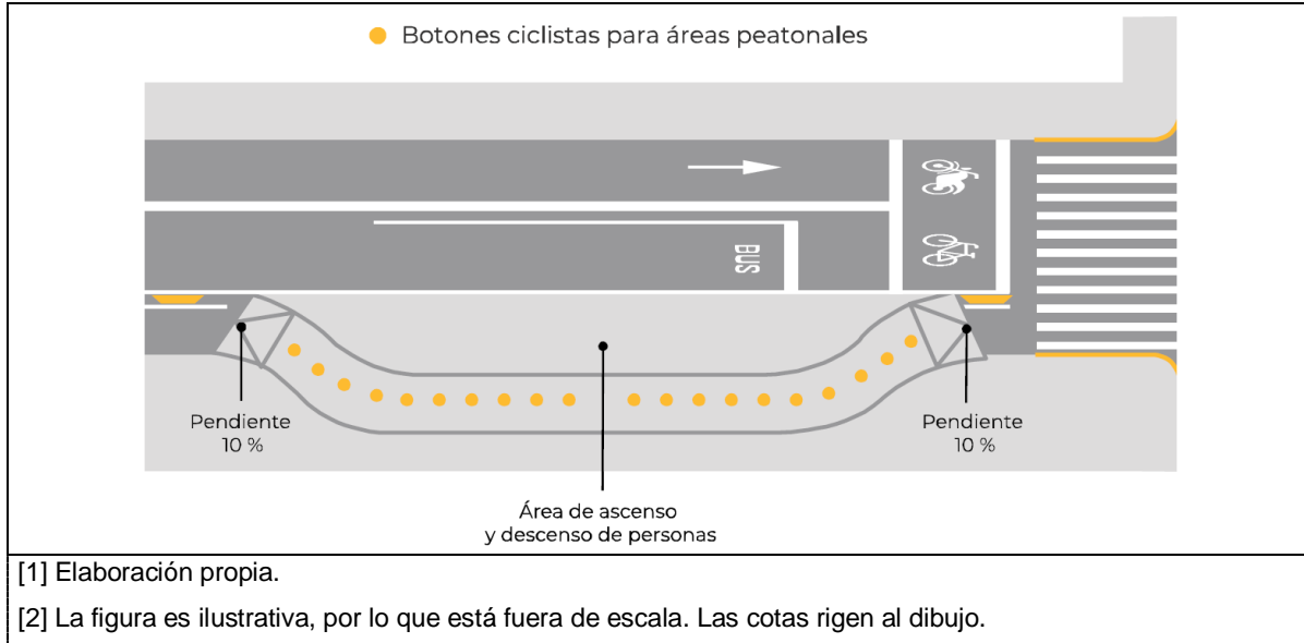
Figura 62.- Parada de transporte público con desvío ciclista [1] [2]
