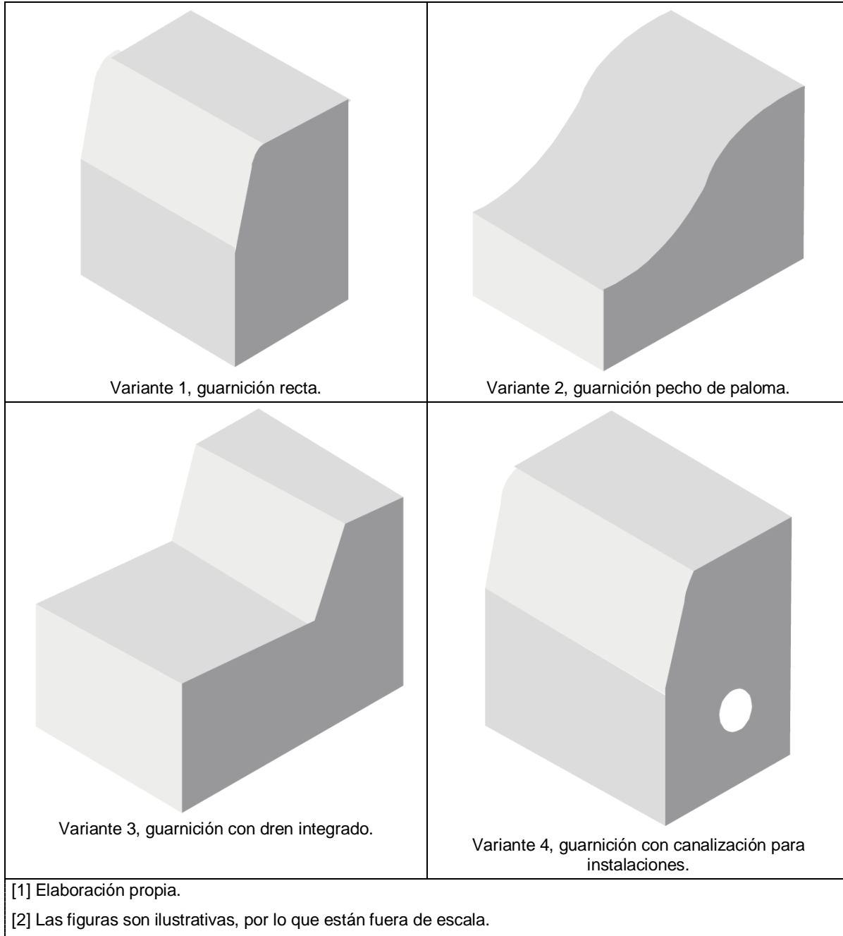
Figura 32.- Tipos de guarniciones [1] [2]
