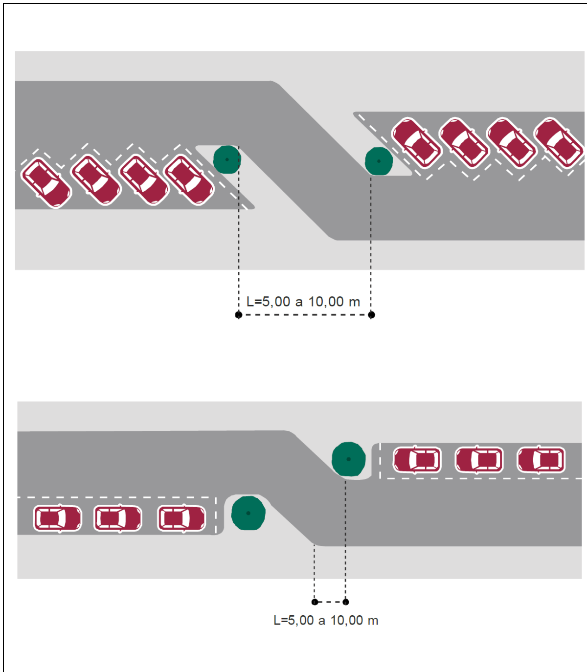
Figura 102.- Zigzag creados por estacionamiento alternado [1] [2]
