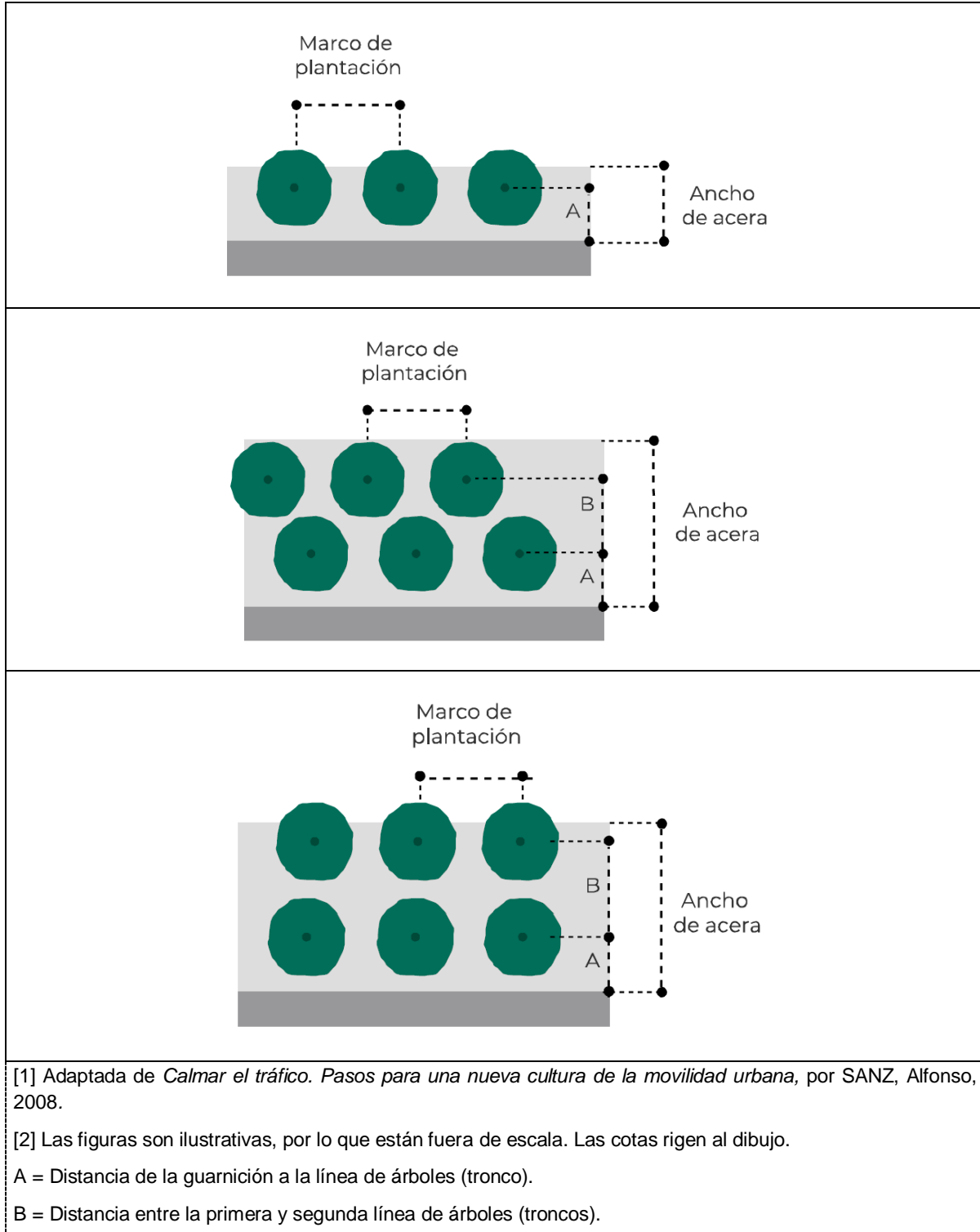
Figura 110.- Dimensiones de referencia para la colocación de árboles en las banquetas. [1] [2]
