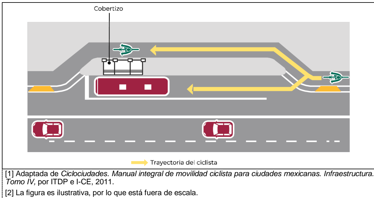
Figura 63.- Parada de transporte público con desvío ciclista y bahía [1] [2]
