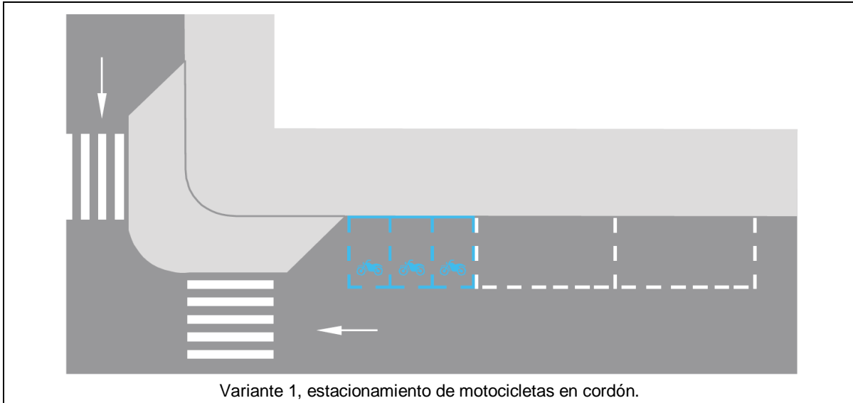
Figura 74.- Disposición de los cajones de motocicletas en relación con la franja de estacionamiento general [1] [2]
