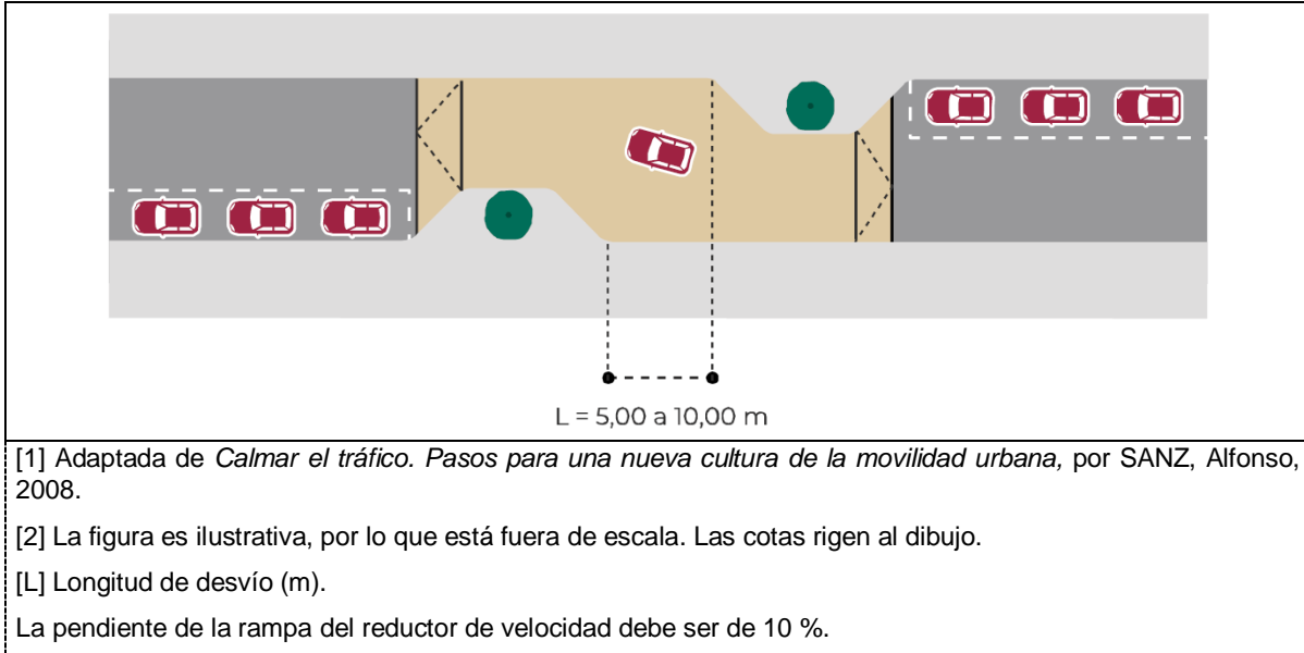
Figura 103.- Zigzag creado por estrechamiento lateral alternativo con meseta [1] [2]
