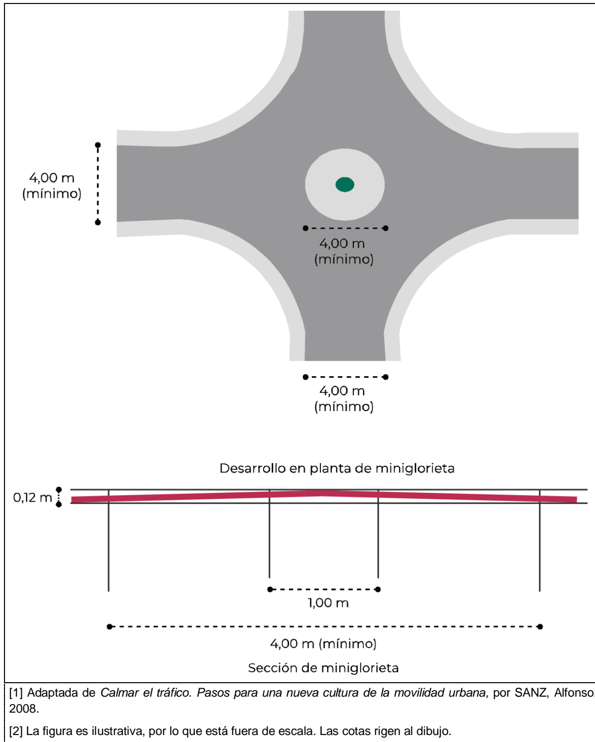
Figura 91.- Geometría de una miniglorieta [1] [2]
