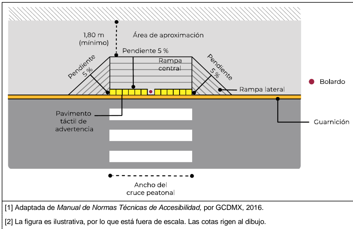
Figura 34.- Rampa con alabeo (planta) [1] [2]
