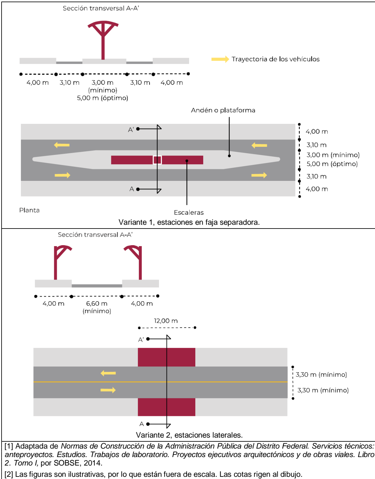
Figura 80.- Estaciones en vías exclusivas para el transporte público de pasajeros [1] [2]
