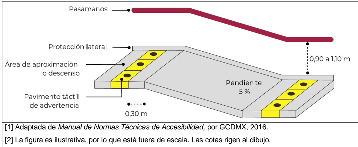
Figura 37.- Rampas en tramos intermedios [1] [2]
