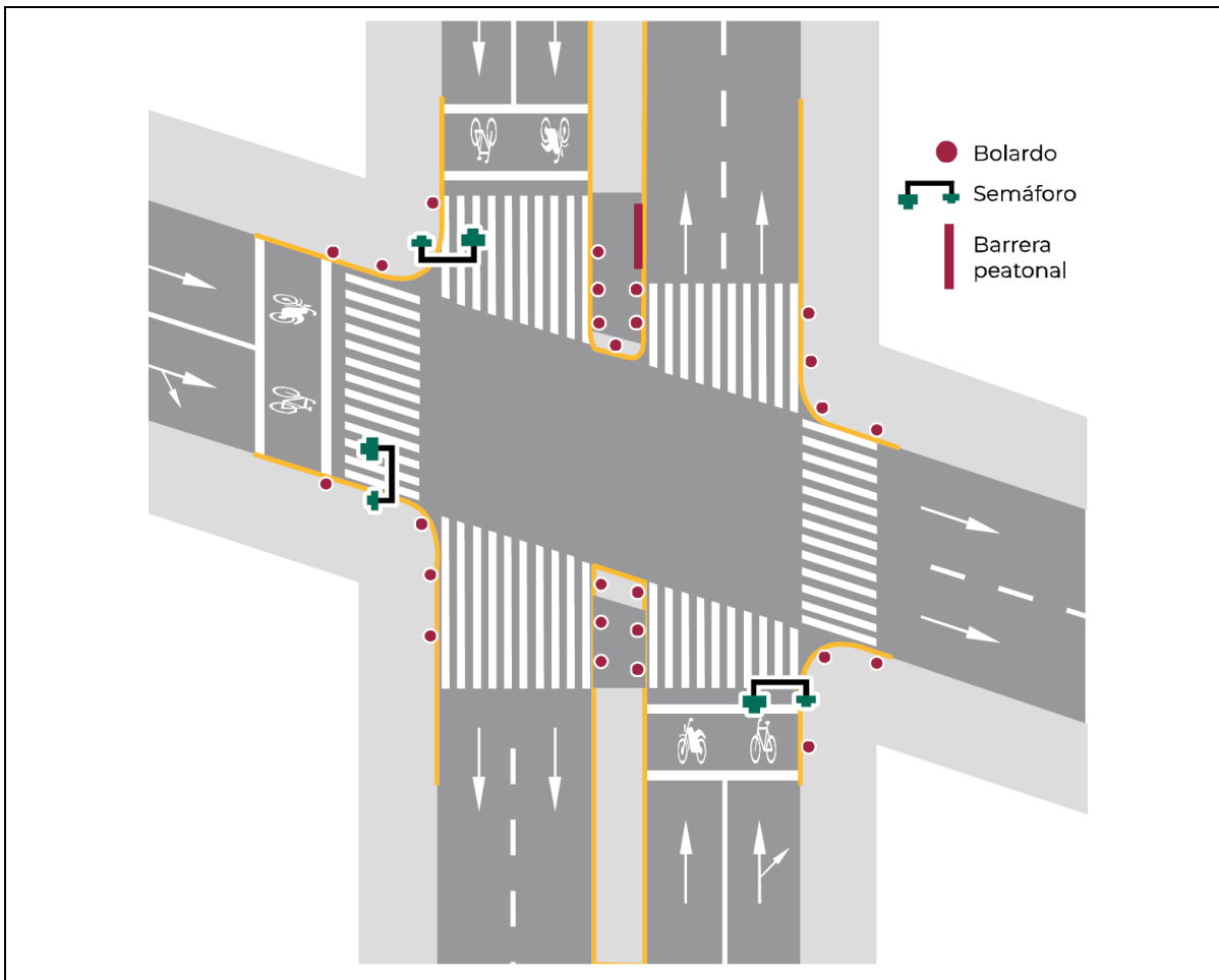
Figura 42.- Cruce peatonal en forma trapezoidal en intersecciones en diagonal [1] [2]
