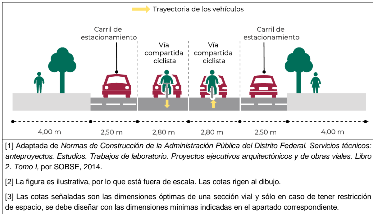
Figura 69.- Calles locales [1] [2] [3]
