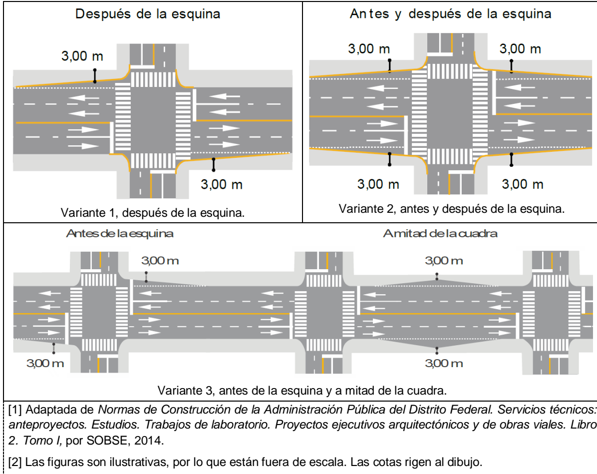
Figura 79.- Diseño mínimo para paradas de autobuses (áreas de transferencia) [1] [2]
