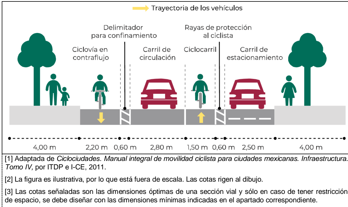
Figura 59.- Perfil tipo de vías ciclistas en contraflujo [1] [2] [3]
