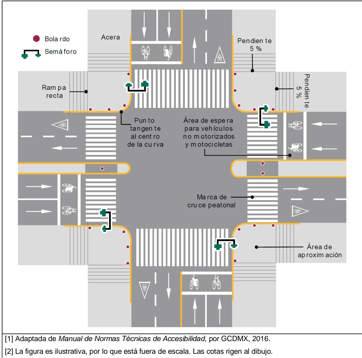
Figura 41.- Emplazamiento de los bolardos (planta) [1] [2]
