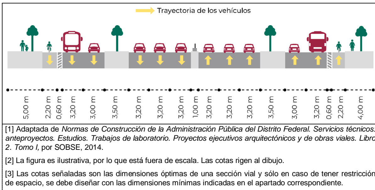
Figura 64.- Vías de circulación continua a nivel [1] [2] [3]
