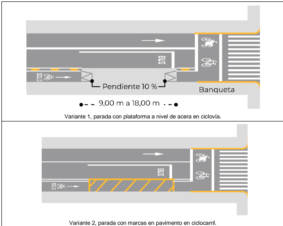
Figura 61.- Tratamientos de paradas de transporte público [1] [2]
