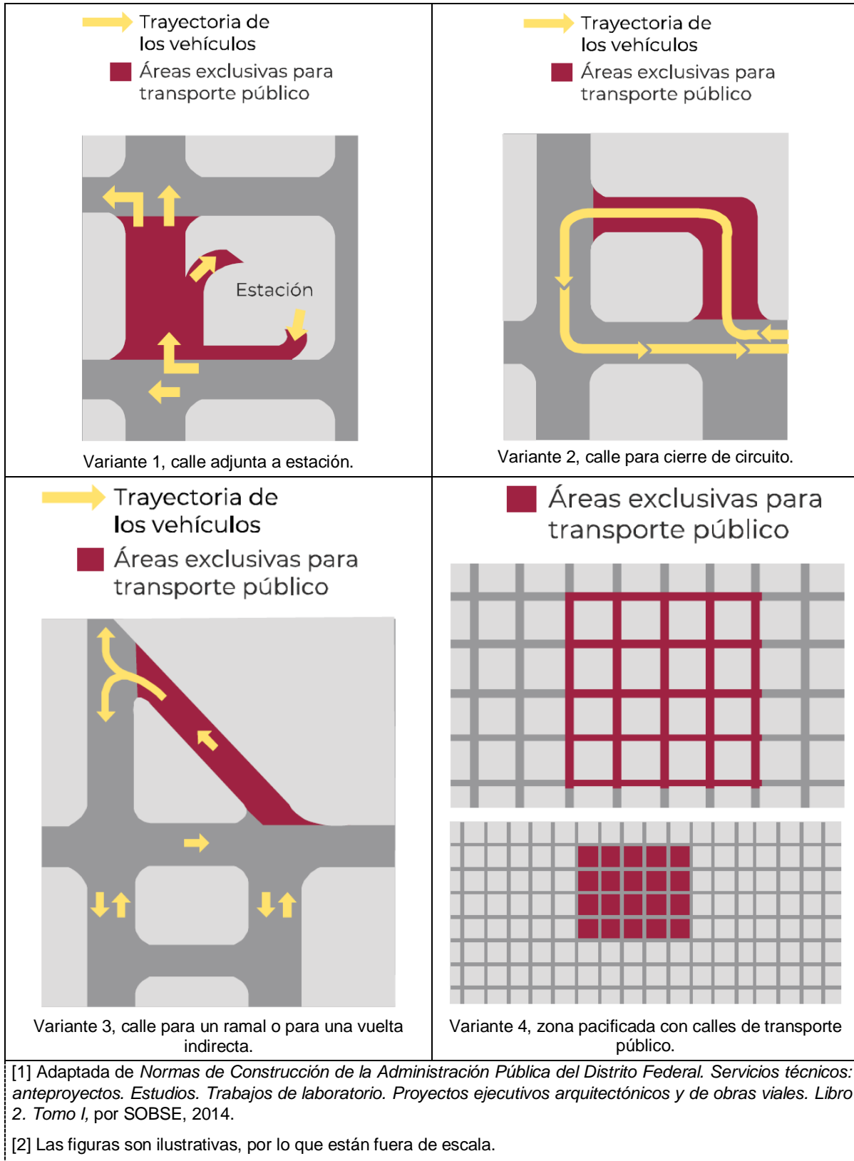
Figura 71.- Casos en los que se requieren calles de transporte público [1] [2]
