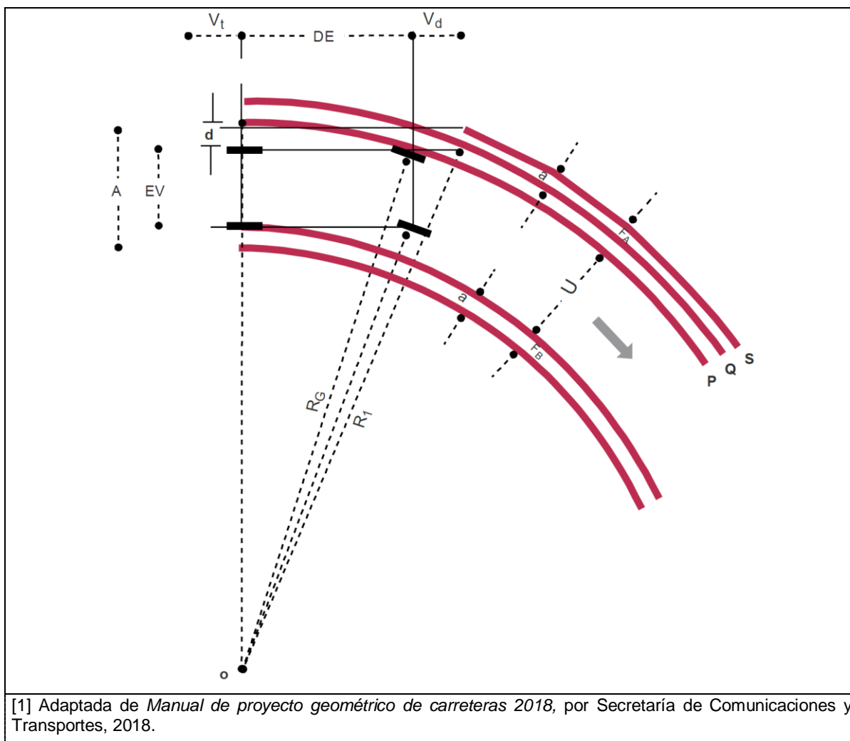
Figura 13.- Ancho en curvas horizontales [1]
