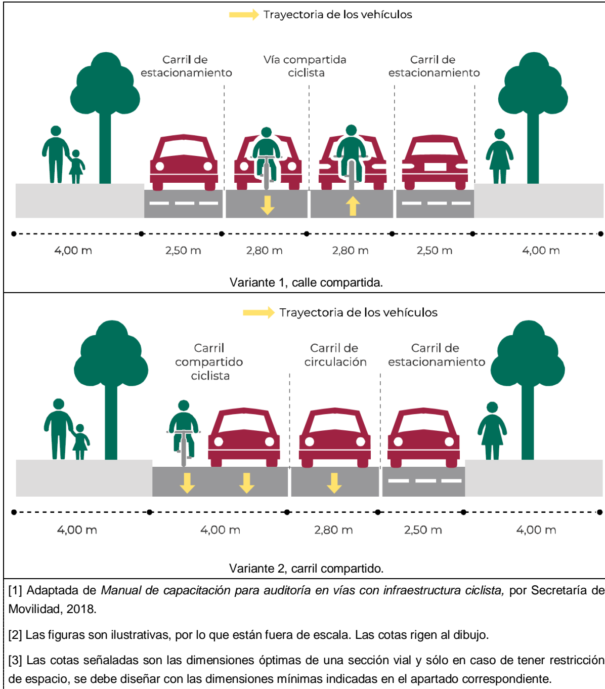
Figura 48.- Perfil tipo de vía ciclista con prioridad de uso [1] [2] [3]
