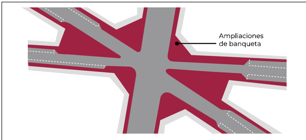
Figura 109.- Modificación geométrica en intersecciones [1] [2]
