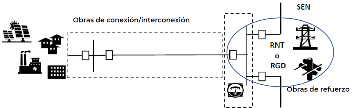
Figura 2.- Punto de Conexión o Interconexión, considerando línea y subestación construidas como instalaciones particulares.
