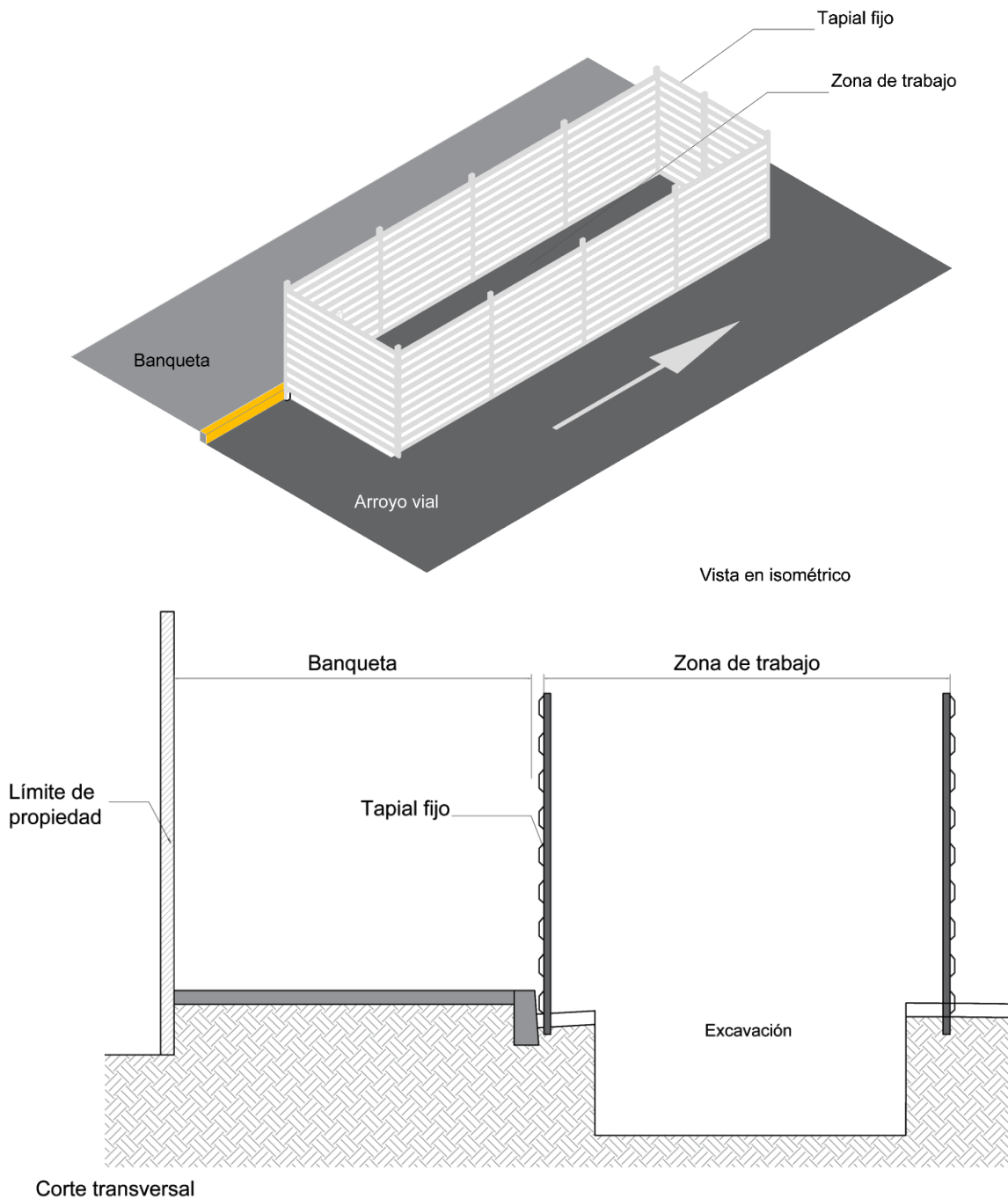
FIGURA 17.- Tapial fijo
