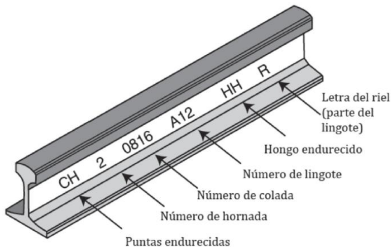
Figura 2 Marcado recomendable del lado interior del riel.
