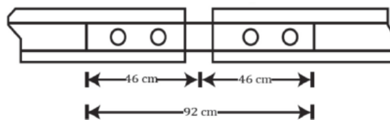
Figura 8 Junta de clase 3 a 5.
