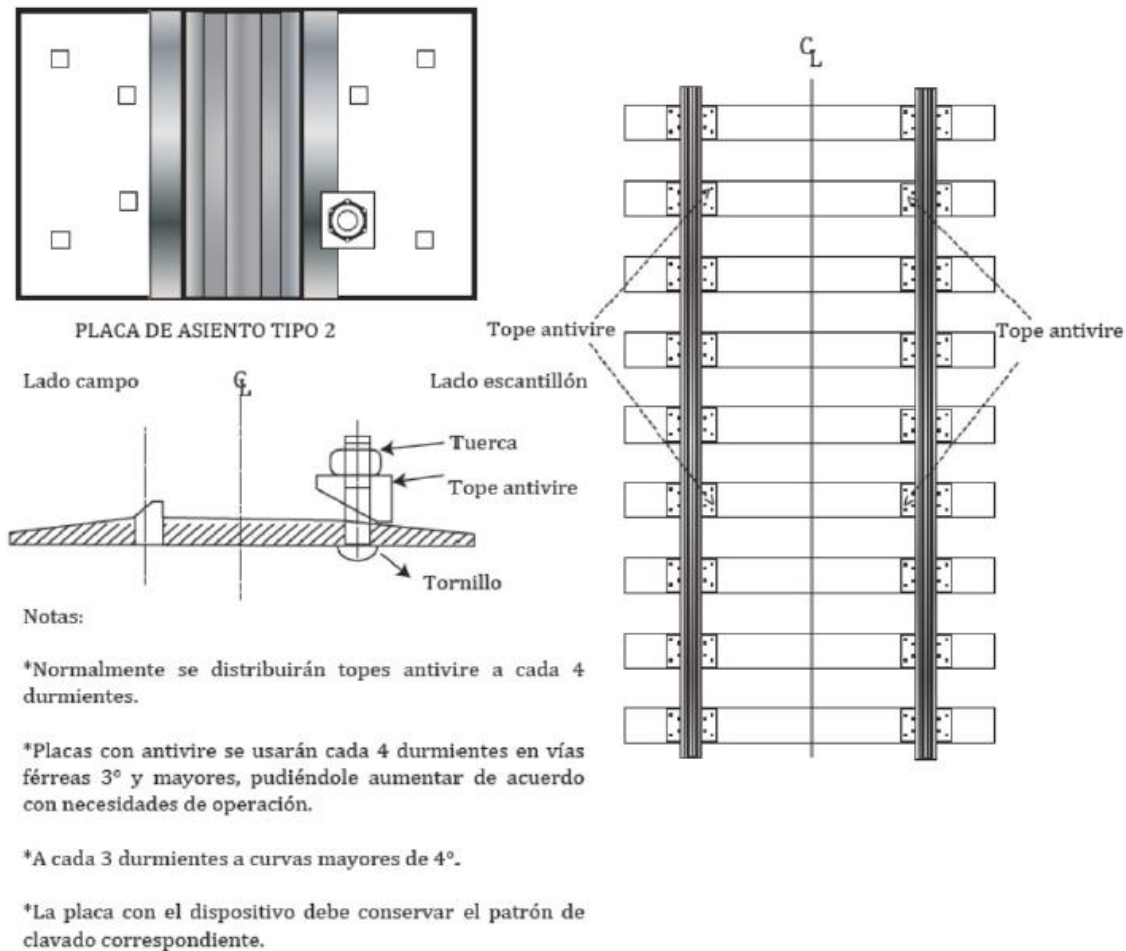
Figura 4 Dispositivos antivire.
