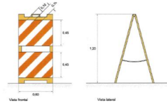
FIGURA 5a. Caballete grande
