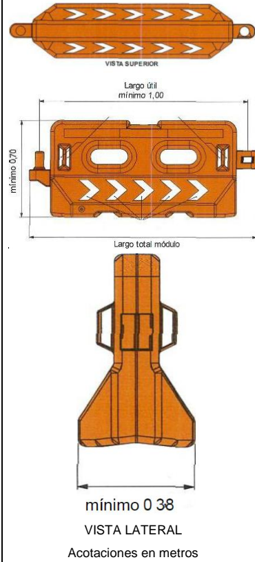
FIGURA 6b.- Barreras canalizadoras Tipo 2.
