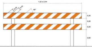
FIGURA 4a.- Barrera fija con postes verticales
