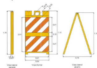
FIGURA 5b. Caballete chico de plástico
