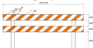
FIGURA 4a.- Barrera fija con postes verticales
