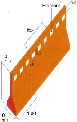
Figura 6ª.- Colocación de las barreras Tipo 1 New Jersey unidas entre si.
