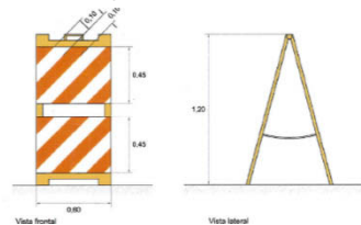
FIGURA 5a. Caballete grande
