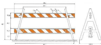
FIGURA 4b.- Barrera fija con postes en forma de "A"
