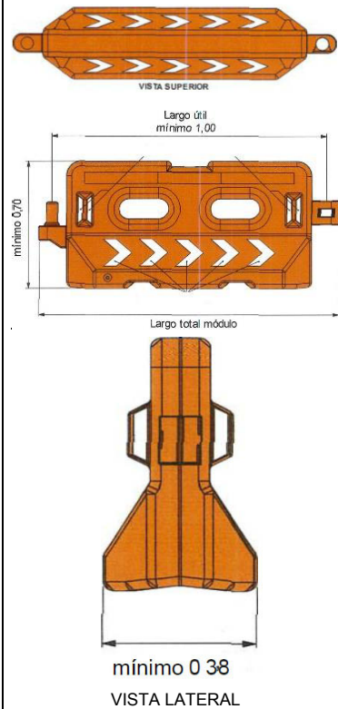
FIGURA 6b.- Barreras canalizadoras Tipo 2.
